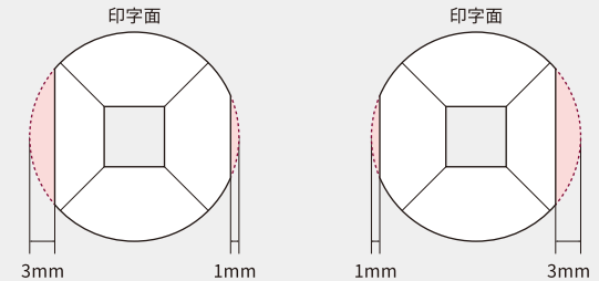
【底面図】
