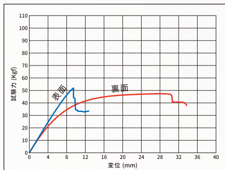
《 三点曲げ機による竹刀ピース破壊耐圧強度比較テスト結果 》
