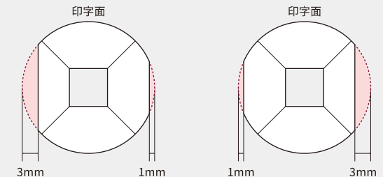
【底面図】
